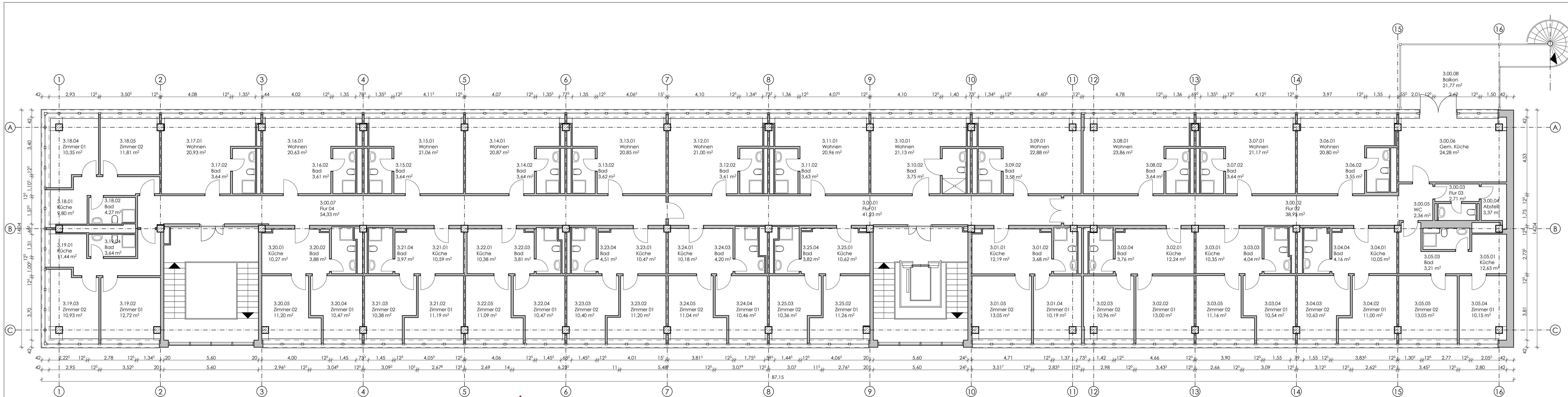
Grundriss 3.OG
